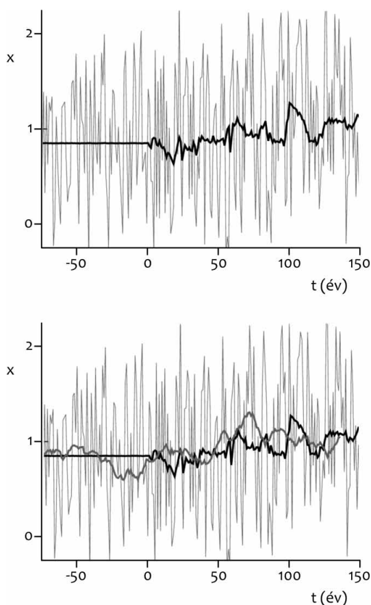
4. ábra • Fent: egyetlen idősor (a nyugati szél erőssége a párhuzamos klímátörténetek egyik elemében [a téli napfordulón], vékony sötétvörös vonal) és a sokaságátlag (vastag fekete vonal) összehasonlítása. Lent: a kiválasztott idősor harmincéves csúszó átlaga a felső kép sötétvörös görbéjére nézve (vastag sötétvörös vonal), az előzőekre rárajzolva.
