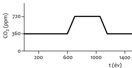
5. ábra • A Planet Simulator klímamodellben használt forgatókönyv (Herein et al., 2016) a \text{CO}_2 -szint változását használja külső gerjesztésként. A változás a 600. évben kezdődik, és az 1150. évben fejeződik be.
