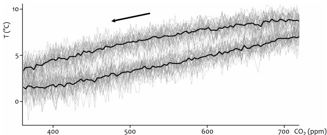
7. ábra • Az előző ábra görbéi a \text{CO}_2 -szint–hőmérséklet ábrázolásban.
