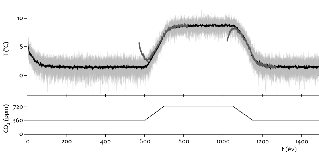
6. ábra • A Pannon-medence felszíni éves átlaghőmérsékletének időfejlődése az alul látható \text{CO}_2 -forgatókönyv következtében a Planet Simulator negyvenelemű sokasága minden egyes tagjában (vékony vonalak), és ezek sokaságátlaga (vastag fekete vonal) (Herein et al., 2016). A t = 0 év kezdőfeltételét t_c = 150 év alatt felejtí el a rendszer: 150 év után éri el a változatlan klímát jellemző konstans értéket. Az 570. és az 1020. évben indított újabb szimulációk átlagértékei (vastag szürke vonalak) szintén kb. ennyi idő után simulnak be az eredeti sokaságátlagba, jelezvén, hogy az eredmény t_c idő eltelte után nem függ a szimulálás indításától.
