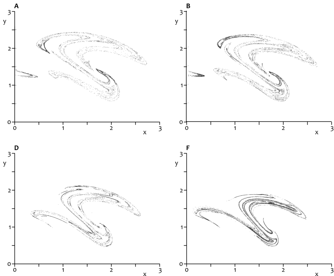
2. ábra • A párhuzamos klímaállapotok tárházat mutató pillanatkép attraktorok (Drótos et al., 2015) az (x,y) , azaz a nyugati szél erőssége - ciklonintenzitás síkon a klímaváltozás kezdetét követő 25., 50., 100. és 150. évben (minden év téli napfordulóján, december 22-én).
