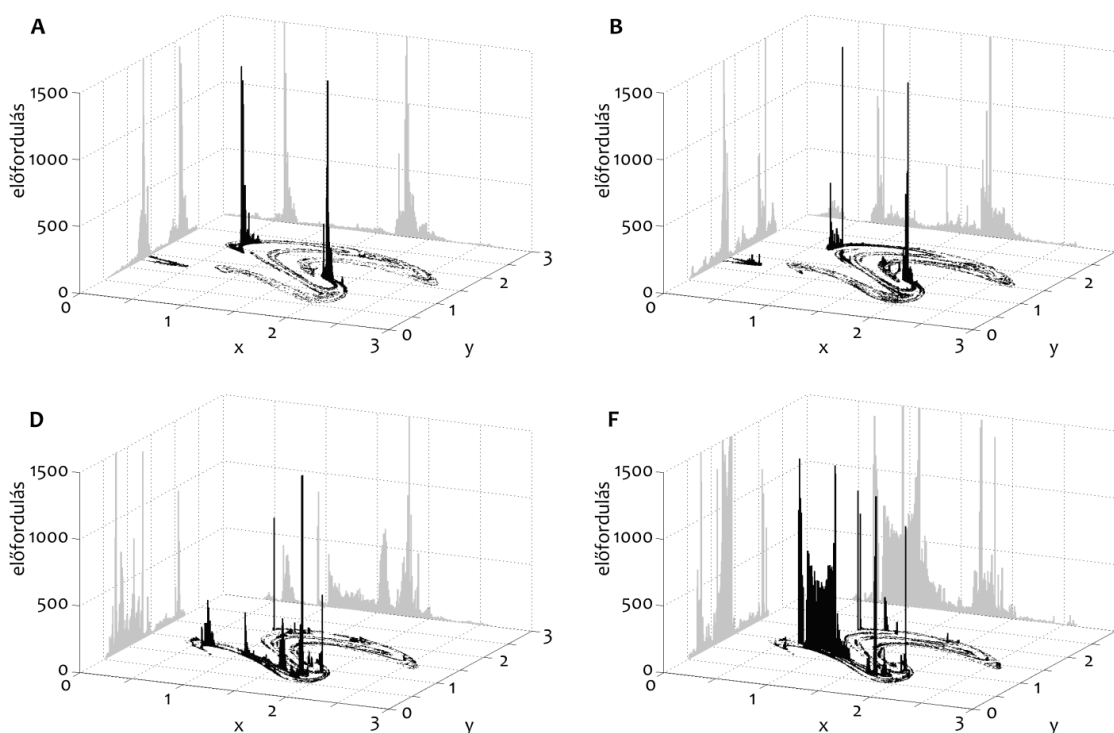
3. ábra • A párhuzamos klímatorténetek által adott természetes eloszlás (Drótos et al., 2015) az (x,y,z = 0) sík felett a klímaváltozás kezdete utáni 25., 50., 88. és 89. évben (minden év december 22-én).
