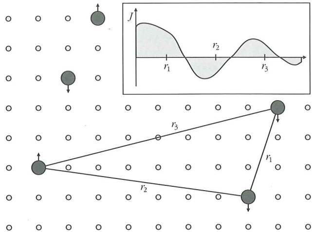
3. ábra. Frusztráció spinüvegekben. Az itt nyilakkal ábrázolt mágneses momentumoknak két lehetséges beállásuk van. A frusztrációt a spinek rendezetlen elhelyezkedése és kölcsönhatási energiájuk oszcilláló csatolási állandója ( J , lásd a mellékábrán) okozza.
